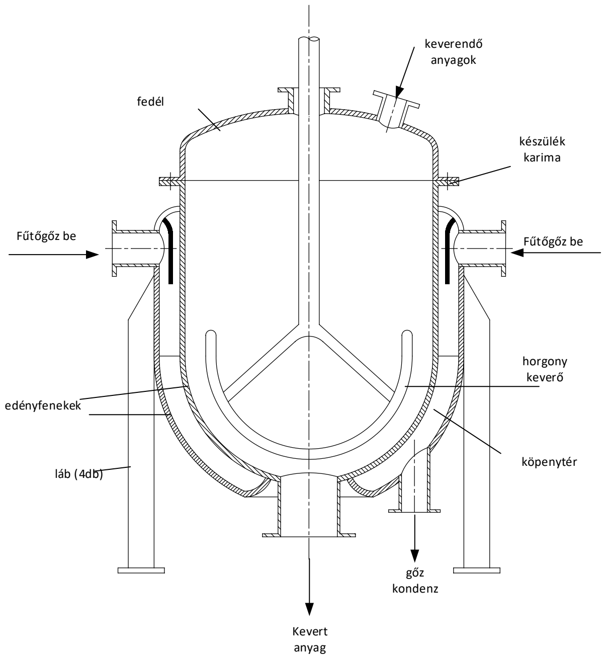
4.1. ábra. Keverős autókláv
